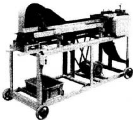
ひも出しロール機の一例（単線）
